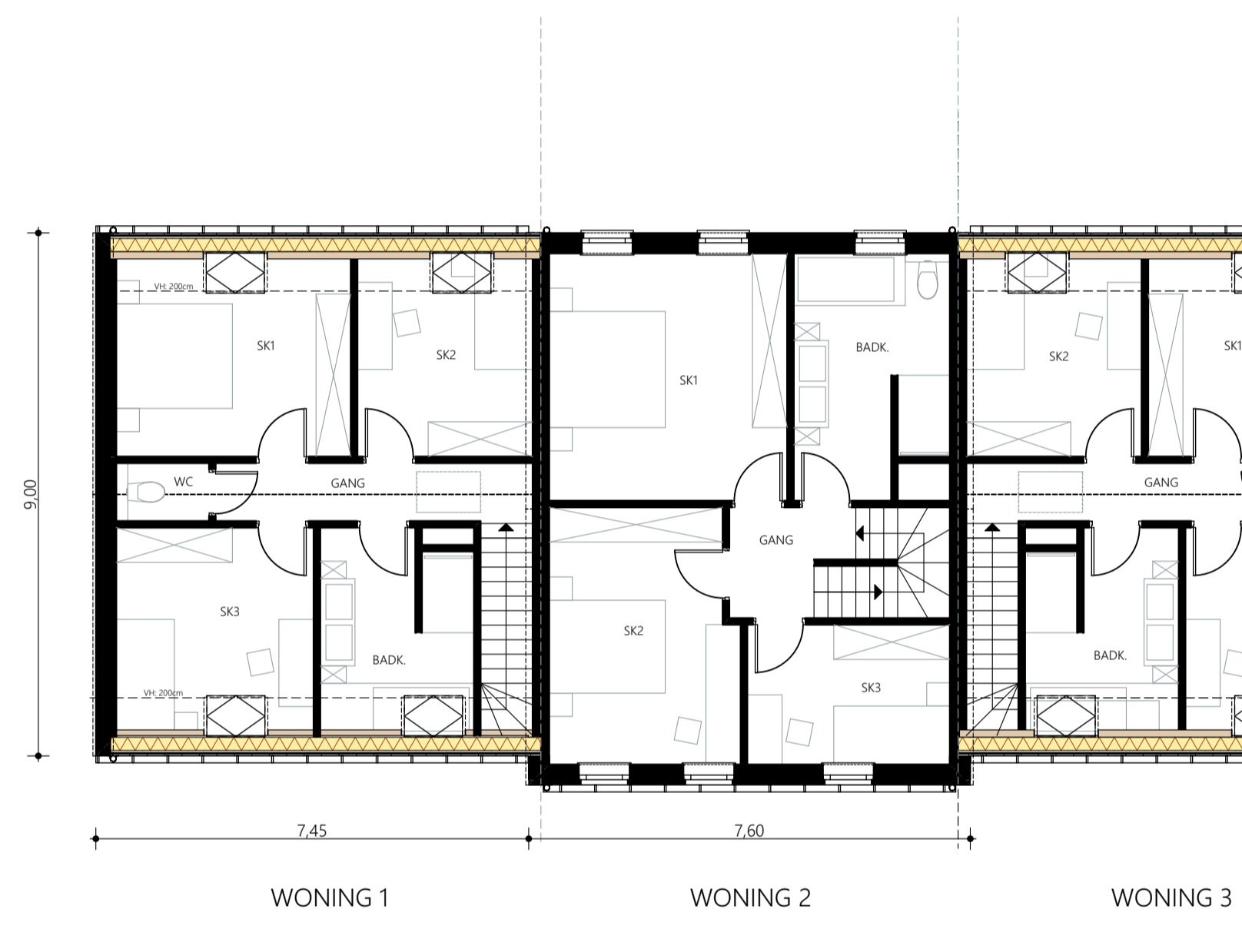
1e VERDIEPING
