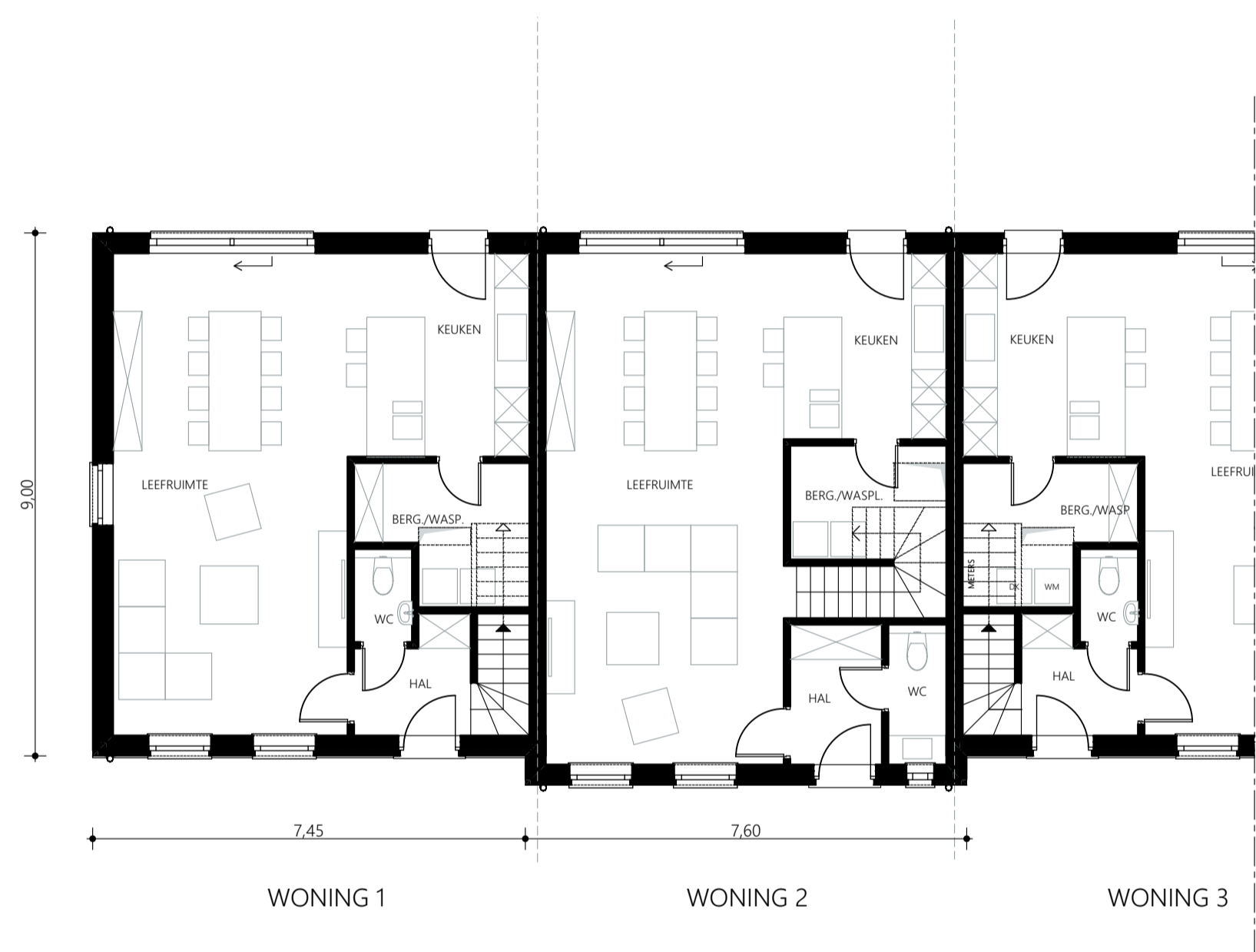
GRONDPLAN
