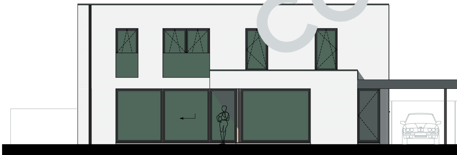
ACHTERGEVEL
